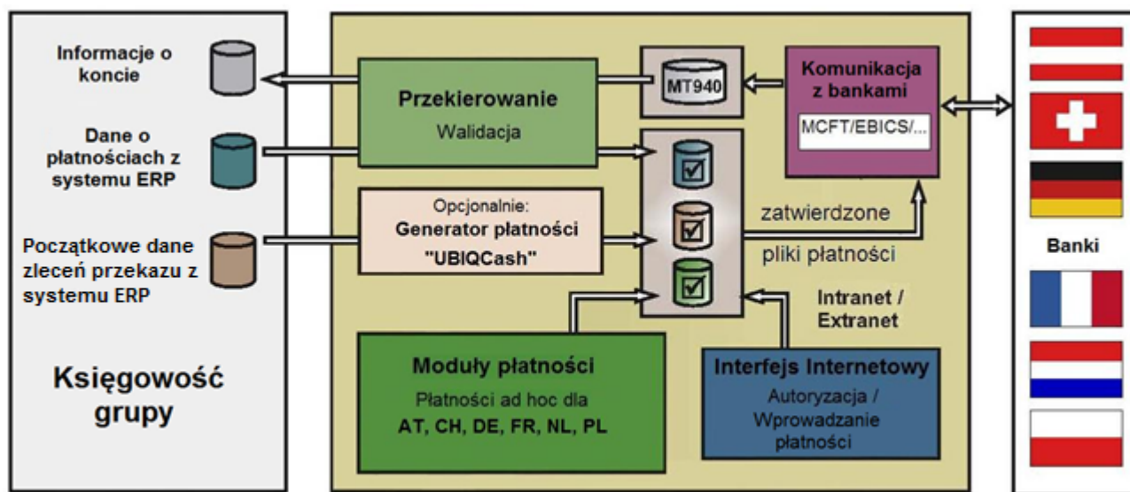
Schemat: MultiCash Transfer jako interfejs pomiędzy ERP a bankami.
